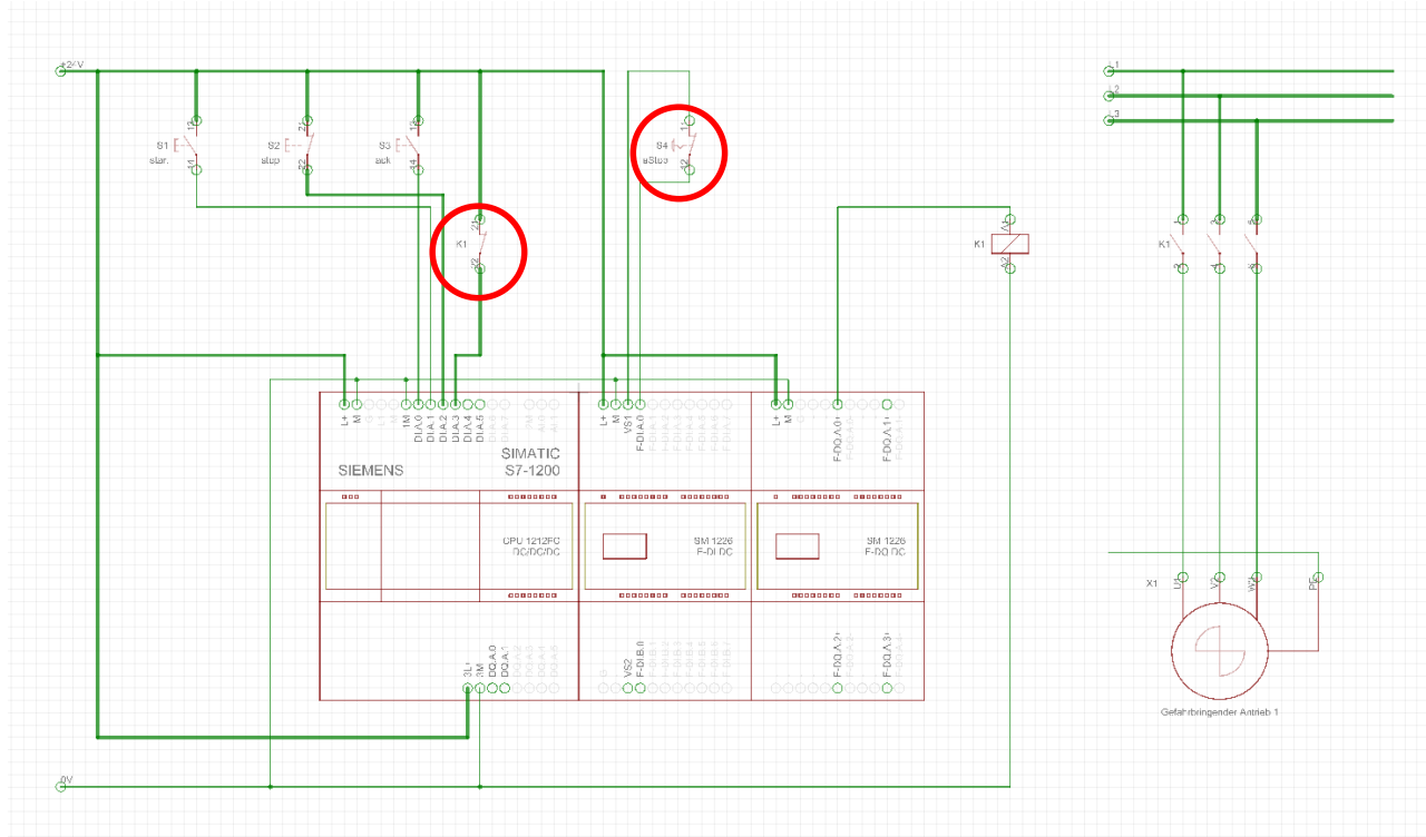
Stromlaufplan SIL 1
